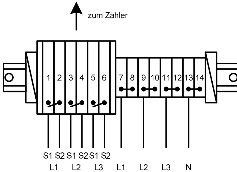
A 1.01 Klemmenleiste für halbindirekte Messungen ohne Datenfernübertragung
